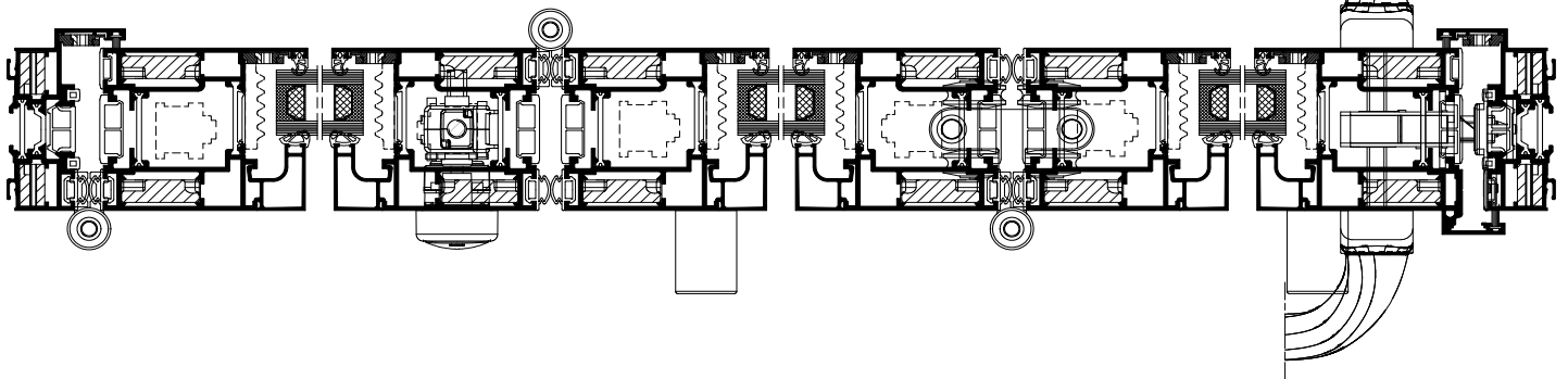
COUPE HORIZONTALE
