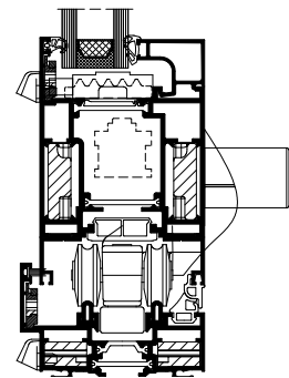
COUPE VERTICALE
